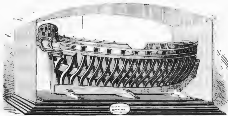
Модель корабля, сдѣланная Петромъ Великимъ, Находится въ Морскомъ музеѣ, въ С.-Петербурѣ.
