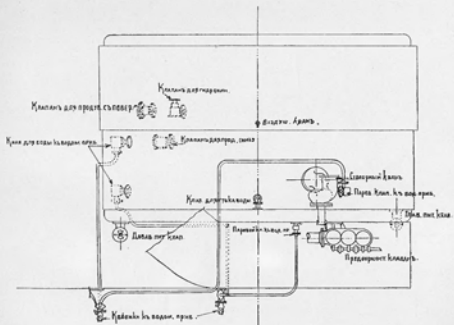
Расположение арматуры
