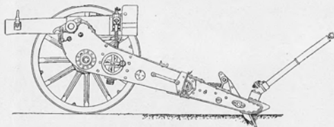
Австр. 7-см. горн. пушка, обр. 99 г.
