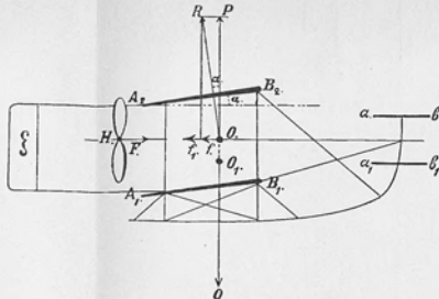
Схема аэроплана бр. Райт.
