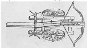
Аркбаллиста.
