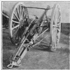
Японское орудіе взятое въ сраженіи на Шахо, въ 1804 г.).
