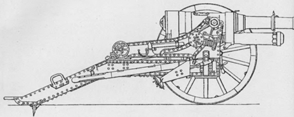
Франц. 120-мм. тяжел. полев. короткая пушка, обр. 90 г.
