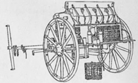
Передокъ герман. 77-мм. полев. пушки.
