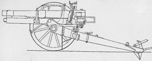
Герм. 77-мм. полев. пушка, обр. 96 г.
