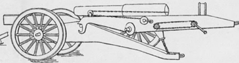
Фриц. 155-мм. тяжел. полев. пушка, обр. 1904 г., перекладывается съ походной повозки (сист. Римальо) на лафетъ.
