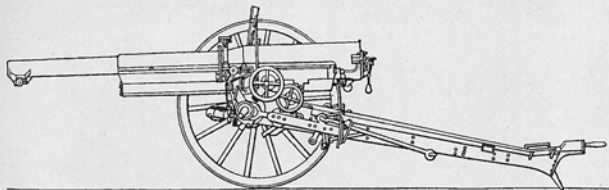
Франц. 75-мм. полев. скоростр. пушка, обр. 1877 г.
