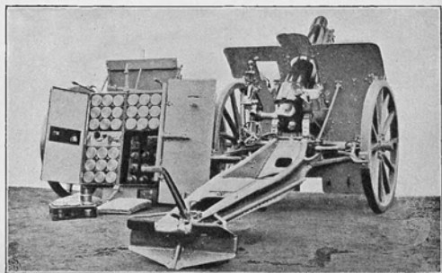
Герман. 10,5-см. легк. полев. гаубица, обр. 98 г.
