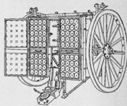
Задн. ходъ зар. ящика франц. полев. скоростр. пушки (на позиціи).
