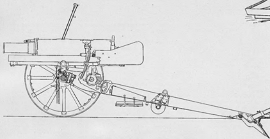
3-дм. гори. скоростр. пушка большой силы, сист. Шнейдера-Дангиса.
