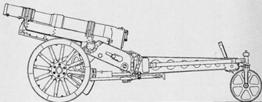
Франц. 65-мм. горн. пушка сист. Дюкре на колесн. передкѣ.
