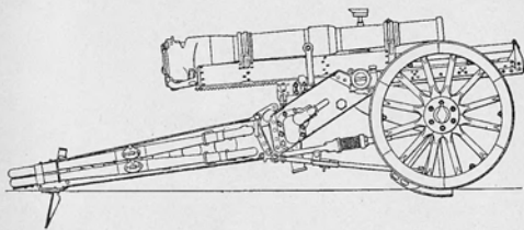
Франц. 65-мм. горн. пушка сист. Дюкре, передъ выстрѣломъ.
