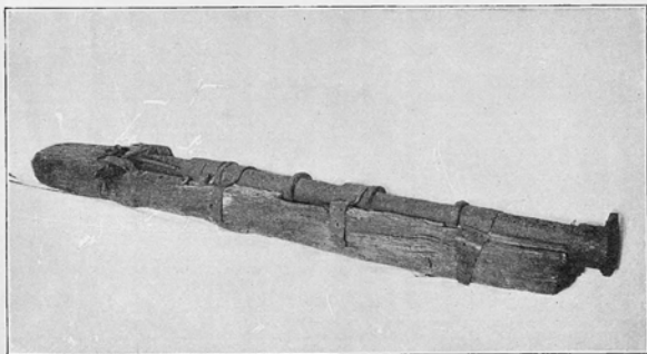
Жельзное, заряжающееся съ казенной части, орудіе начала XV вѣка.
