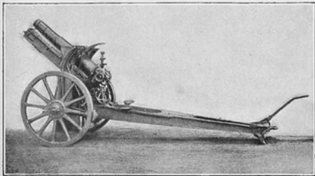
Швейц. 12-см. тяжелая полев. гаубица.
