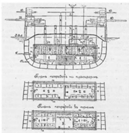
СХЕМАТИЧЕСКІЙ ЧЕРТЕЖЪ АРТИЛЛЕРІЙСКАГО ПОГРЕБА НА СУДАХЪ ФЛОТА.
