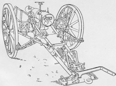
Австр. 10-см. полев. легк. гаубица, обр. 99 г.
