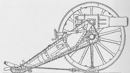
Англ. 5-дм. полев. гаубица, обр. 96 г.
