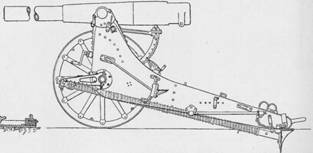
Герм. 10,5-см. пушка тяжел. полев. арт-ии.
