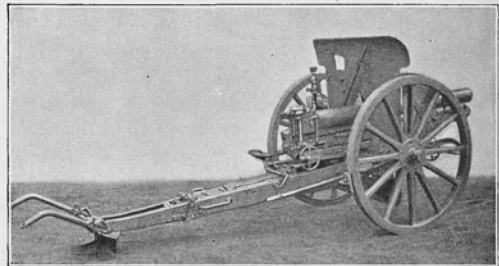
Нидерландск. 75-мм. полев. полуавтоматич. пушка для индійск. островн. колоній.
